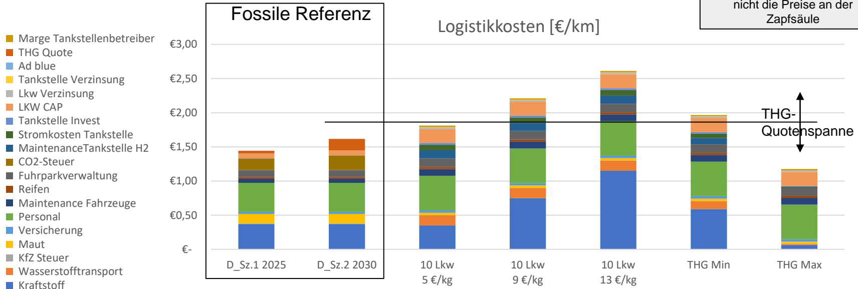
Eigene Berechnung: Förderung: 80% Mehrkosten Fahrzeug; Tankstelle 45% CAPEX; Fahrzeugpreis: Diesel: 80k€; FCEV: 385k€
