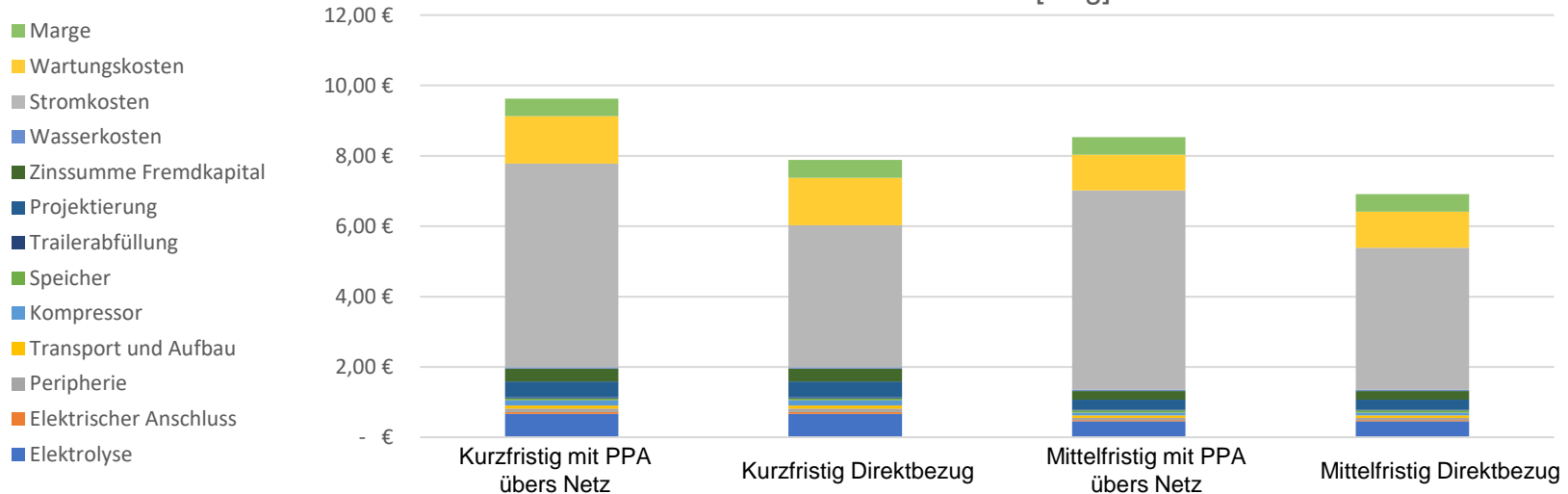
Wasserstoffkosten [€/kg]
